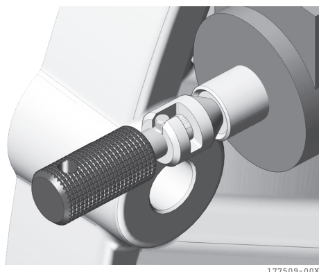
Figure 8 Aucun solénoïde activé (point mort)
