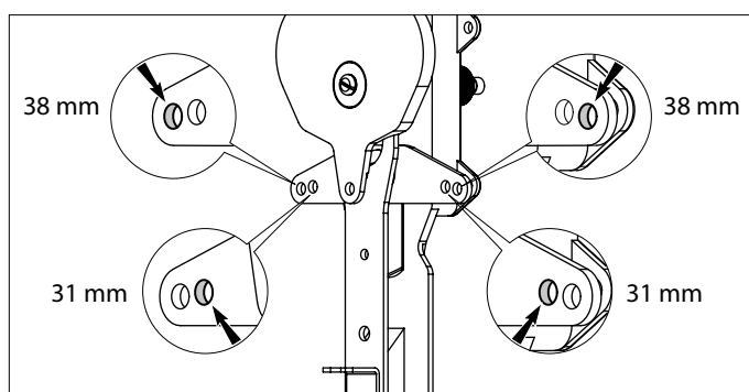
Course du câble de boîte de vitesses
