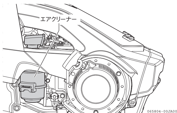
図 2-17 エアクリーナー
