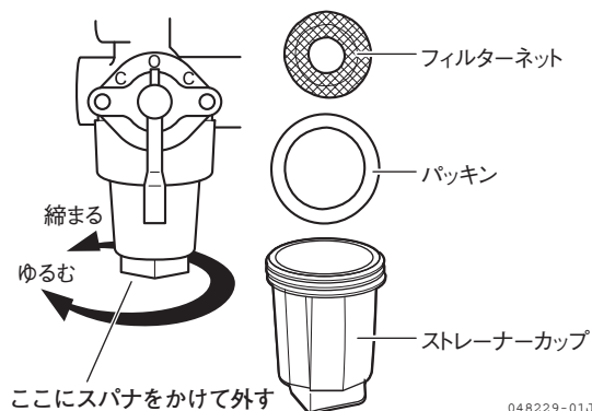
図 4-22 燃料コシ器エレメント
