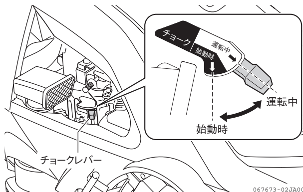
図 2-14 チョークレバー
