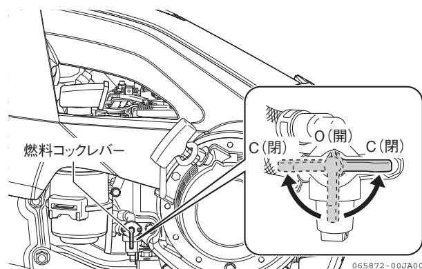
図 2-38 燃料コックレバー
