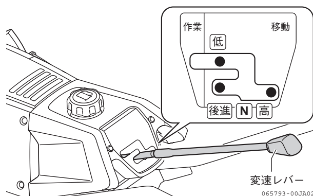
図 2-26 変速レバー（標準・Z仕様）
