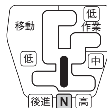
図 2-20 変速レバー N位置（Z2仕様）
