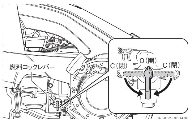
図 2-18 燃料コックレバー
