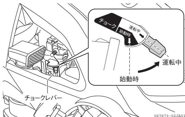
図 2-25 チョークレバー
