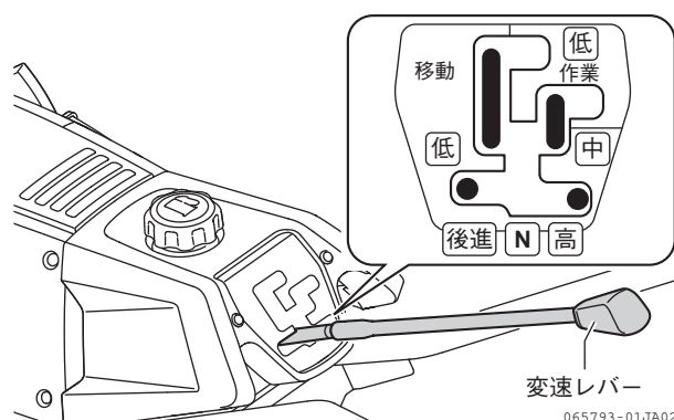
図 2-27 変速レバー（Z2仕様）
