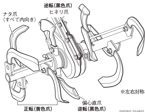
図 4-38 爪の取付方向
