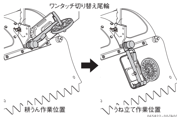
図 3-17 耕うん・うね立て
