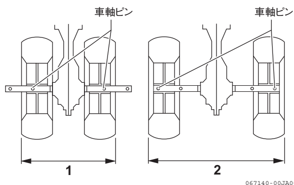
図 3-10 タイヤ取付幅変更
