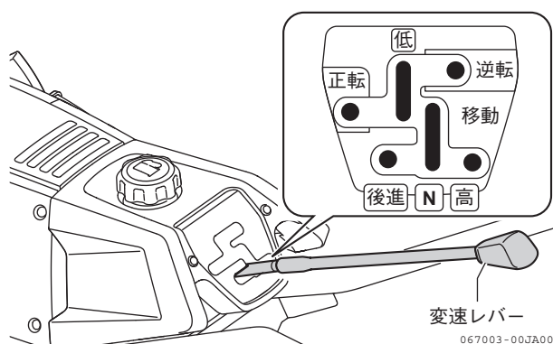
図 2-8 変速レバー (UV仕様)
