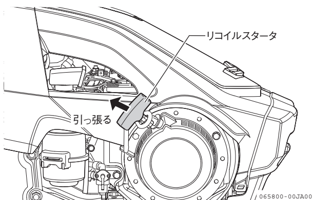
図 2-24 リコイルスタータ
