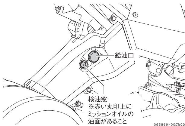
図 4-17 点検のしかた
