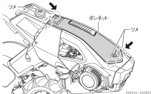
図 4-42 ボンネット
