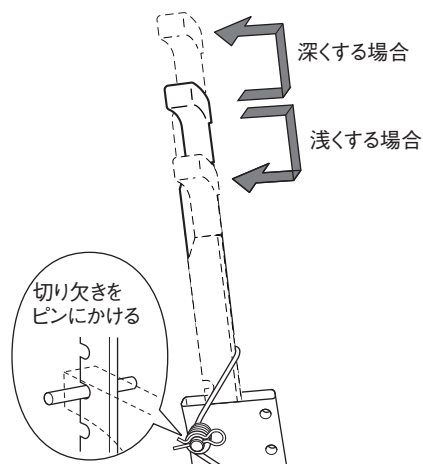
図 3-11 耕深調節棒
