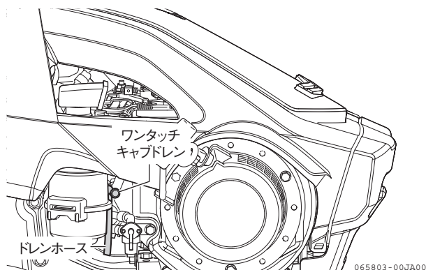
図 2-16 ワンタッチキャブドレン
