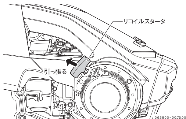
図 2-13 リコイルスタータ
