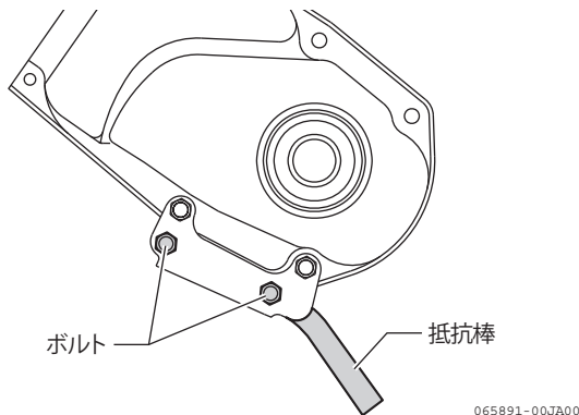
図 4-41 抵抗棒
