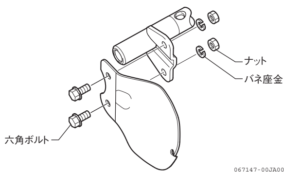
図 4-34 爪交換（ハイブリッド爪）
