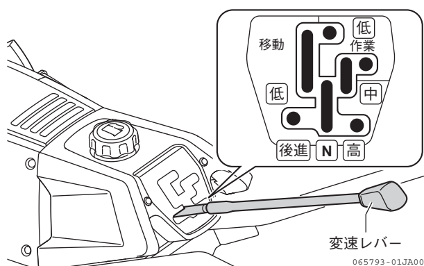
図 2-7 変速レバー（Z2仕様）
