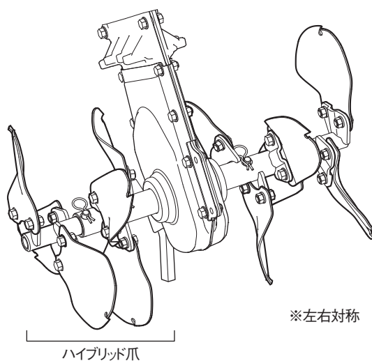
図 4-39 爪の取付方向
