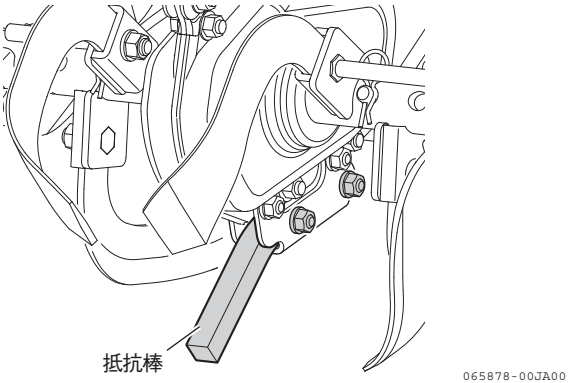
図 4-29 抵抗棒
