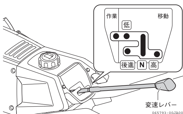
図 2-6 変速レバー（標準・Z仕様）
