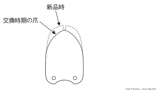
図 4-31 耕うん爪の摩耗 (ハイブリッド爪)
