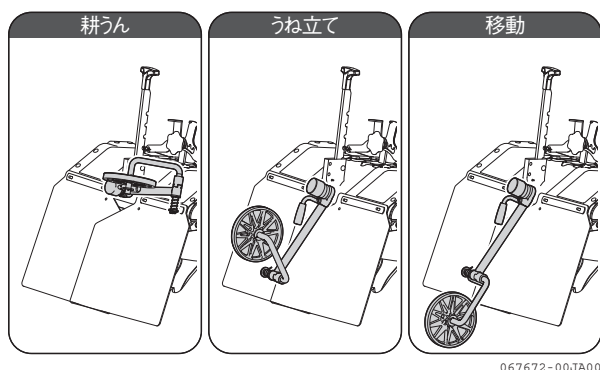
図 2-12 ワンタッチ切り替え尾輪 (UV仕様)
