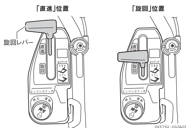
図 2-5 旋回レバー
