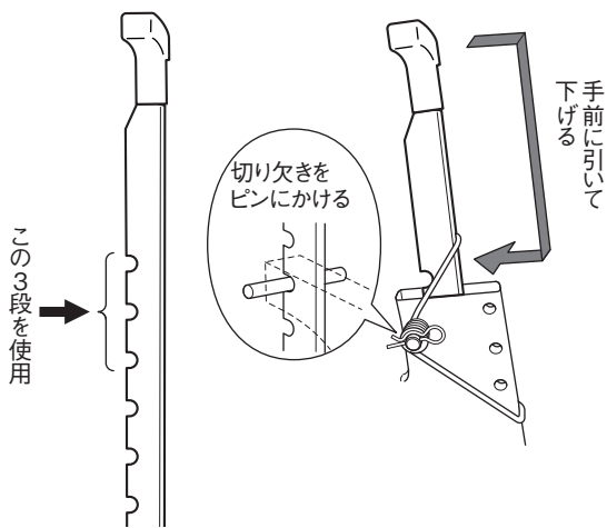
図 3-16 耕深調節棒（下）
