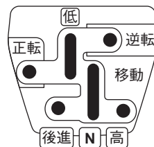
図 2-31 変速ガイド（UV仕様）
