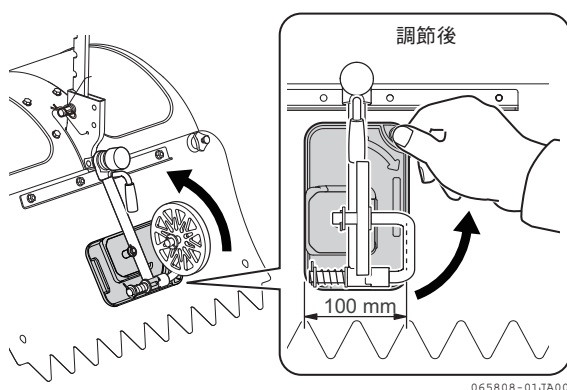
図 3-21 うね立て（溝底幅切り替えプレート縦）
