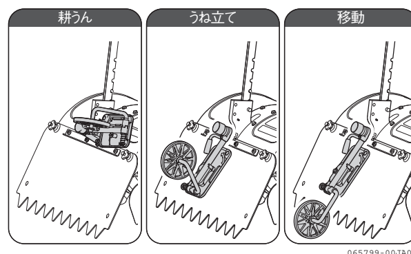
図 2-11 ワンタッチ切り替え尾輪 (標準・Z・Z2仕様)
