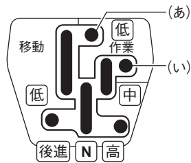
図 2-30 変速ガイド（Z2仕様）
