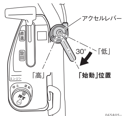
図 2-22 アクセルレバー
