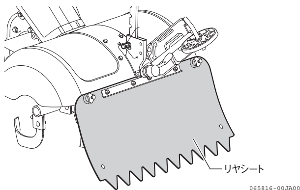
図 3-12 リヤシート
