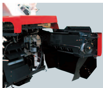
●カッターオープン
