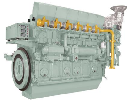
<左:2 段過給システム搭載エンジン「6EY26W」、右:船用デュアルフューエルエンジン「6EY26DF」>
