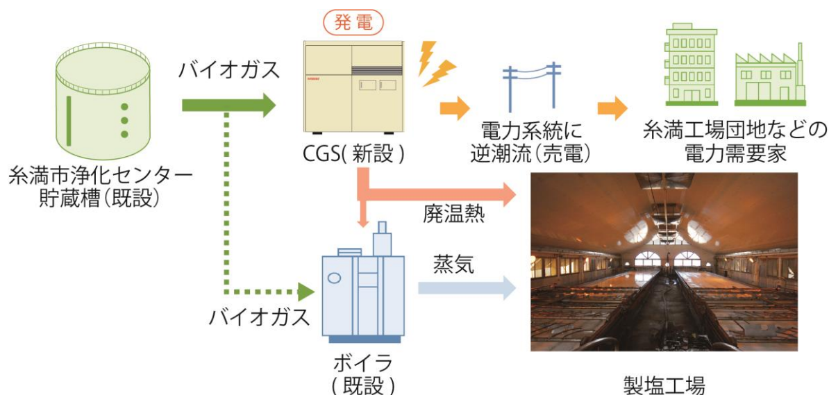
<参考：導入設備のフロー>
