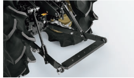
リンケージドロワー ロアリンクに装着できるドロワーヒッチです。
