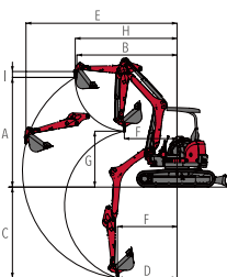
ViO30-7 標準仕様(標準アーム0.09m 3 バケット付き)
