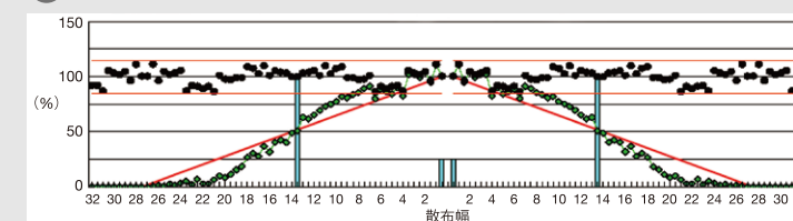
図1 散布量チャート 縦軸：散布量／横軸：散布幅(27m幅)
