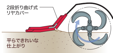
2段折り曲げ式仕様
