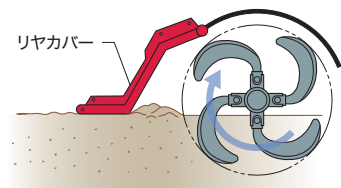
標準リヤカバー
