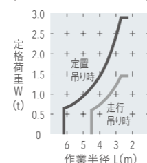
標準仕様 (標準アーム0.37m/バケット付き)
