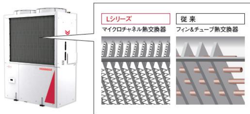
<マイクロチャネル熱交換器>
