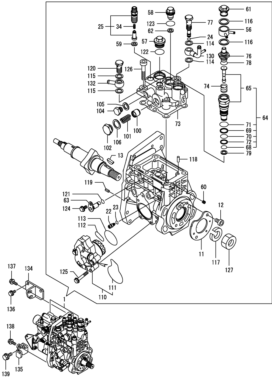
OCNP6-M06220 ชุดเครื่องยนต์ Fig.13. ชุดปั๊มน้ำมันเชื้อเพลิง
