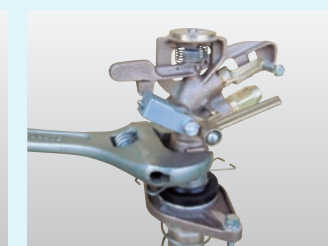
インターナル上部、下部 取り外し状況
