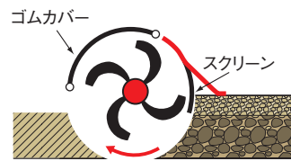
回転方向 上が細かく、下が粗い、理想的な2層構造
