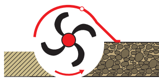
一般ロータリーの耕起断面
