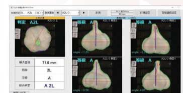
5面計測カラーカメラ(AI画像処理機能付)
