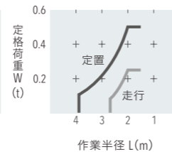
クイックヒッチ仕様 (標準アーム0.08m 3 バケット付き)
