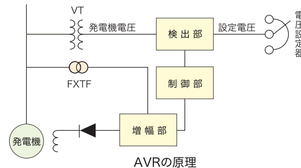
AVRの原理
