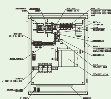
ZPC2-5S1内部構造図
