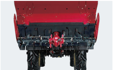
延長爪軸キット (センターロータリー用) 1B1500-29011-2 ※片側100mm
