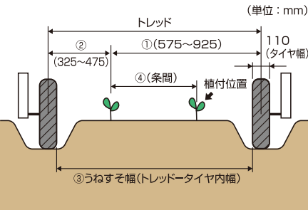
※図は、タイヤ位置が出荷状態(左右のタイヤは内向き)になっています。
