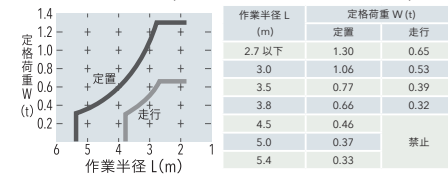
ViO55-6Cクイックヒッチ仕様(標準アーム0.16m 3 バケット付き)
