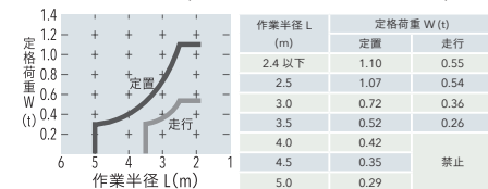
ViO45-6Cクイックヒッチ仕様(標準アーム0.14m 3 バケット付き)
