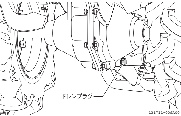
図 4-19 交換のしかた（ドレンプラグ）
