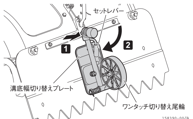
図 3-6 尾輪（うね立て作業）
