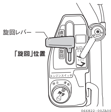
図 2-27 旋回レバー（旋回）
