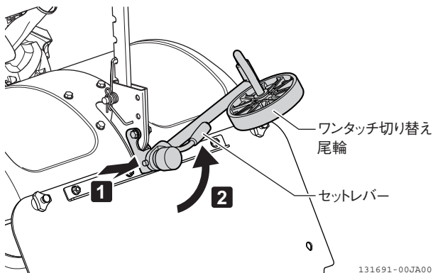
図 3-3 尾輪（耕うん作業）
