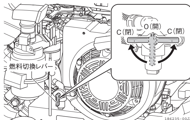
図 2-34 燃料切換レバー
