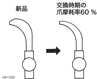
図 4-29 耕うん爪の摩耗
