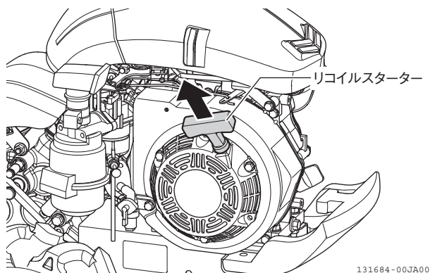
図 2-20 リコイルスターター
