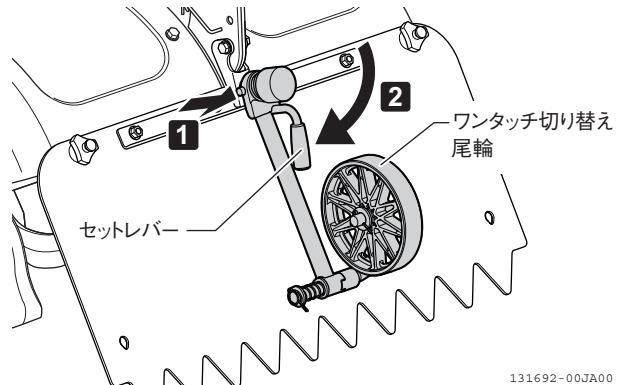
図 3-5 尾輪（うね立て作業）
