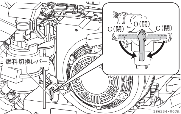
図 2-16 燃料切換レバー
