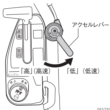
図 2-31 アクセルレバー
