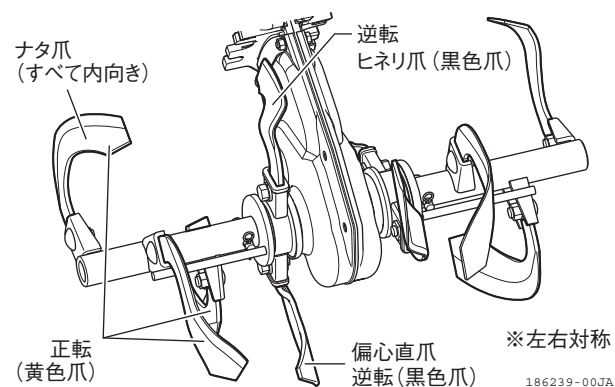
図 4-32 爪の取付方向 (YK400CR,ZL・ZLE仕様)
