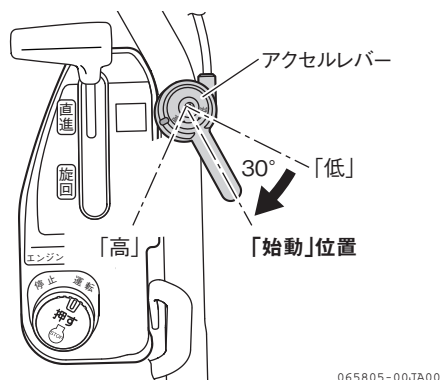
図 2-18 アクセルレバー
