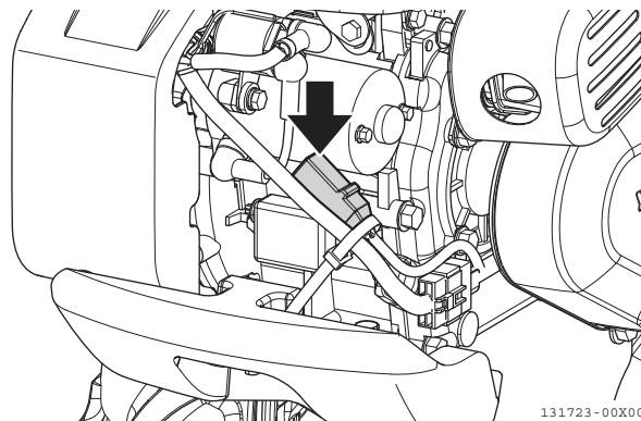
図 4-40 ヒューズ
