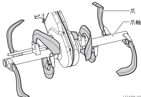
図 4-1 爪と爪軸
