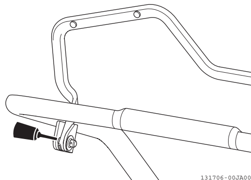
図 4-8 主クラッチレバー
