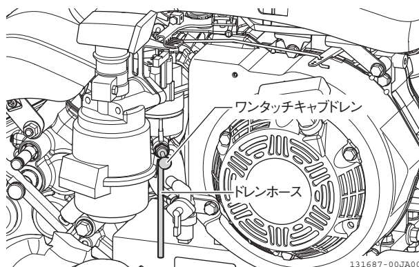
図 2-14 ワンタッチキャブドレン
