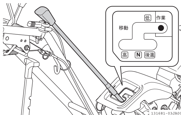
図 3-15 変速レバー
