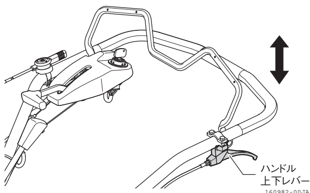
図 2-8 ハンドル上下レバー
