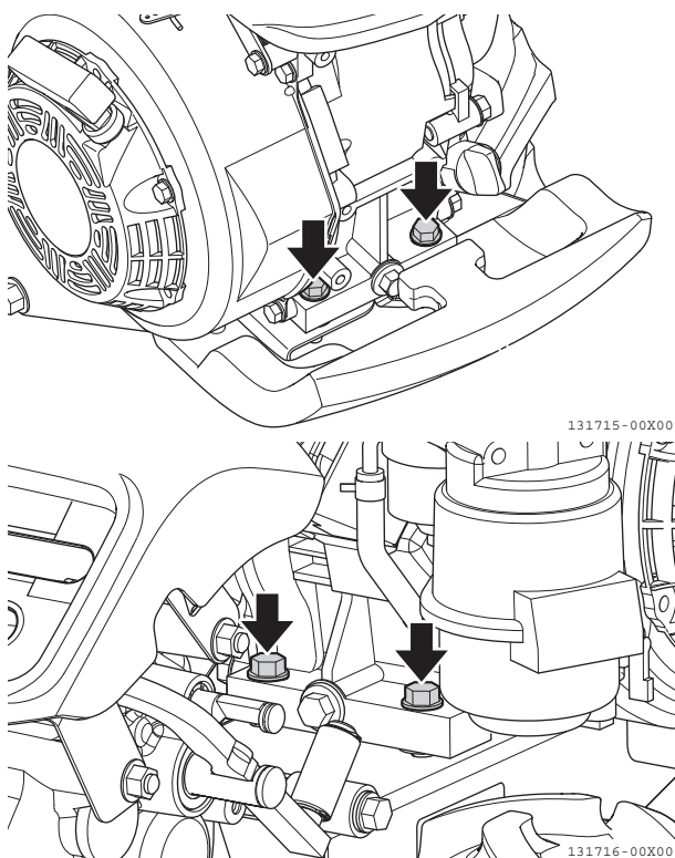
図 4-26 エンジンボルト
