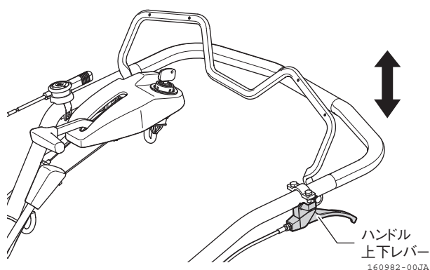
図 3-2 ハンドル上下レバー
