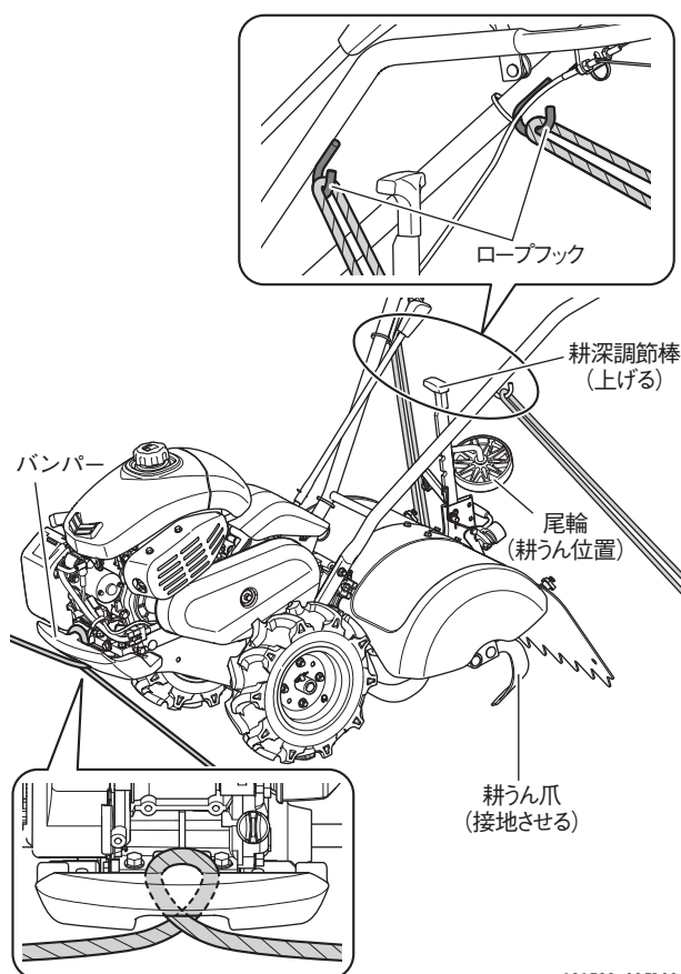
図 6-1 ロープ固定
