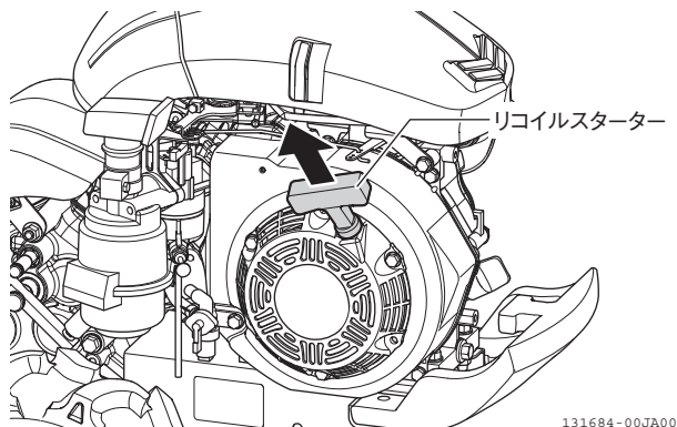
図 2-11 リコイルスターター
