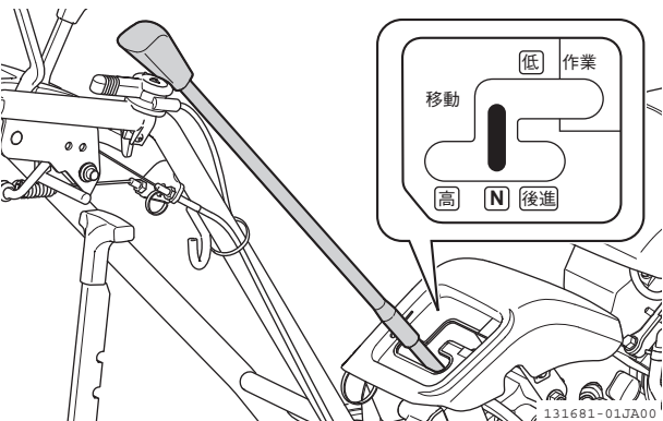
図 2-17 変速レバー
