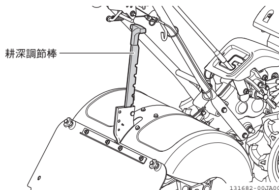
図 2-9 耕深調節棒
