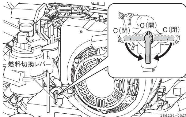
図 2-13 燃料切換レバー
