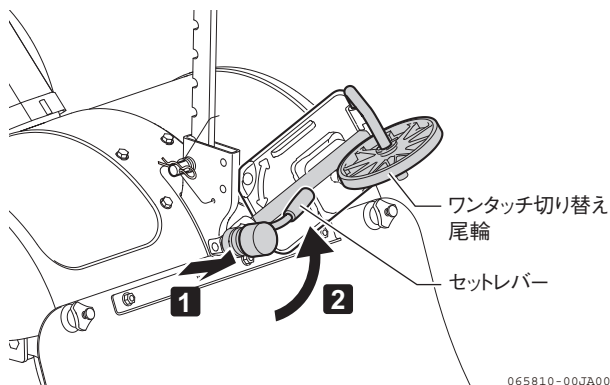
図 3-4 尾輪（耕うん作業）
