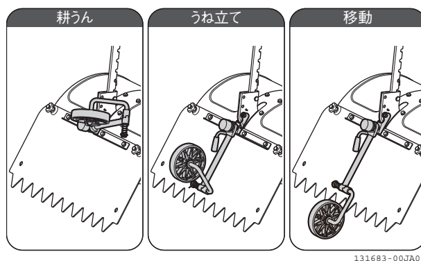
図 2-10 ワンタッチ切り替え尾輪
