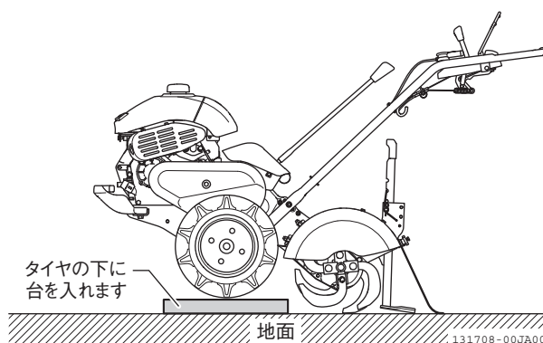
図 4-15 エンジン水平
