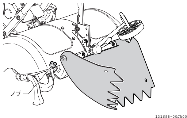
図 3-19 うね立て (リヤシート)
