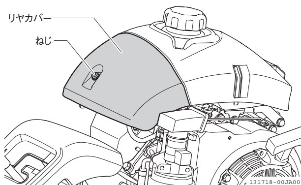
図 4-34 リヤカバー
