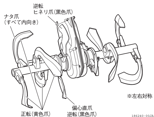
図 4-33 爪の取付方向
