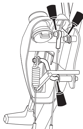
図 4-7 主クラッチレバー・旋回レバー支点・ 主クラッチワイヤ支点
