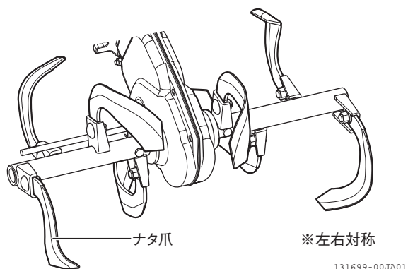
図 4-31 爪の取付方向 (YK400CR,標準仕様)
