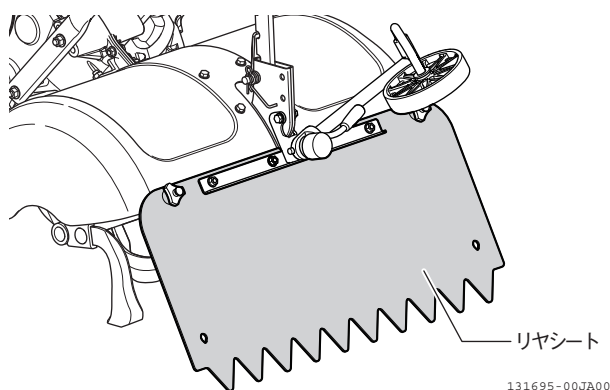
図 3-13 リヤシート
