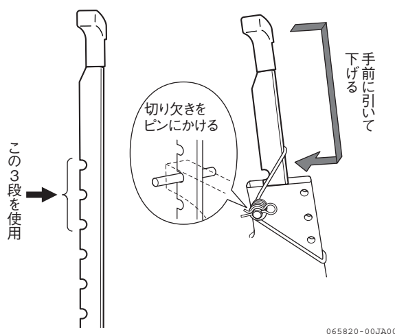
図 3-16 耕深調節棒 (下)
