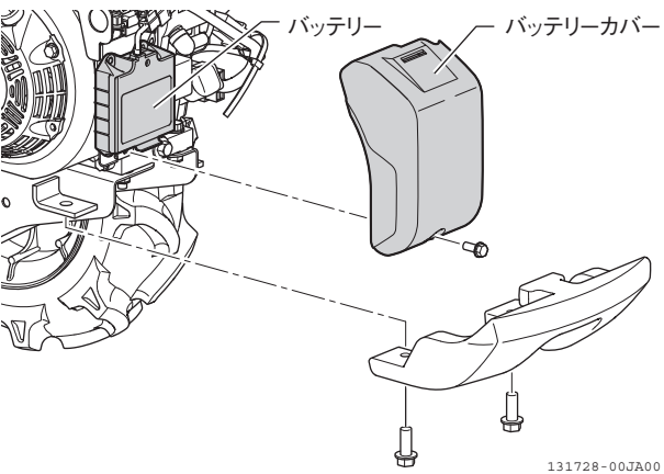
図 4-39 バッテリー
